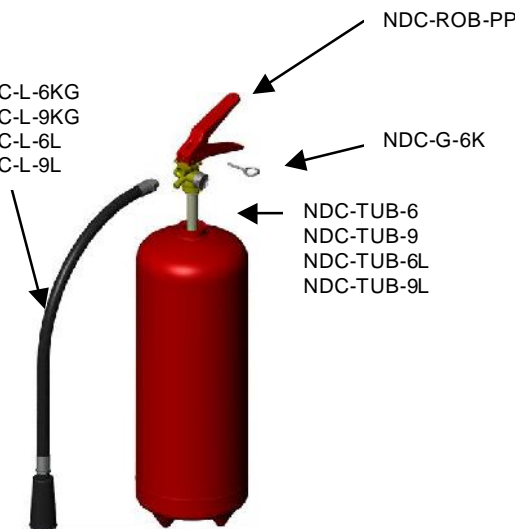
Extincteur CPP-Max 6 / 9 litres Eau avec Additif
