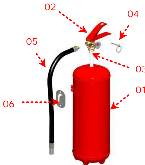
Extincteur Manofeu 6 / 9kg Poudre
